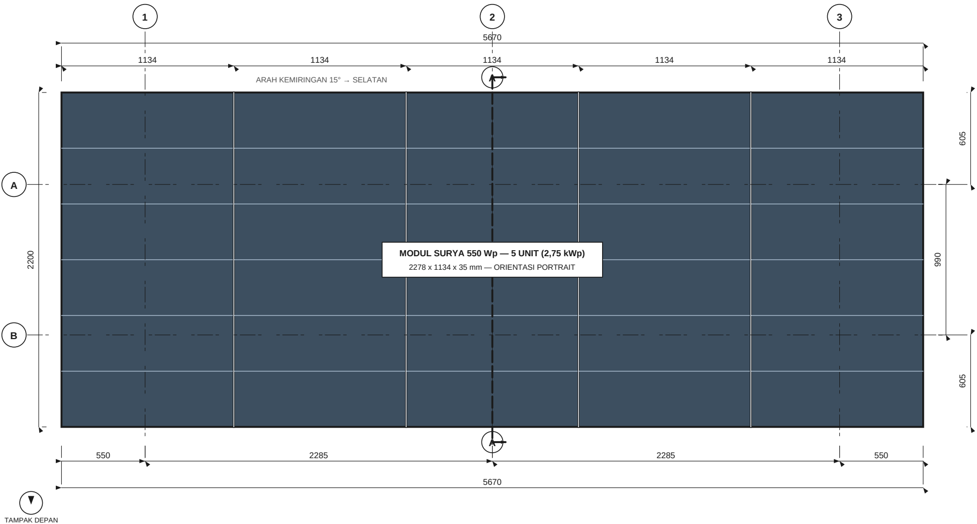
TAMPAK ATAS SKALA 1 : 25
